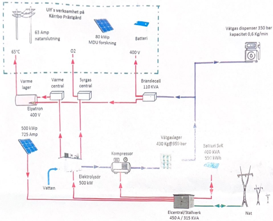
Figur 1. Principbild energisystem.
