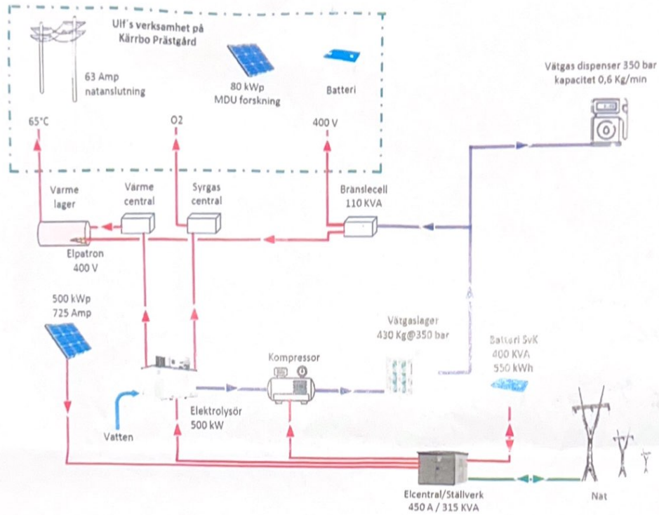
Figur 1. Principbild energisystem.
